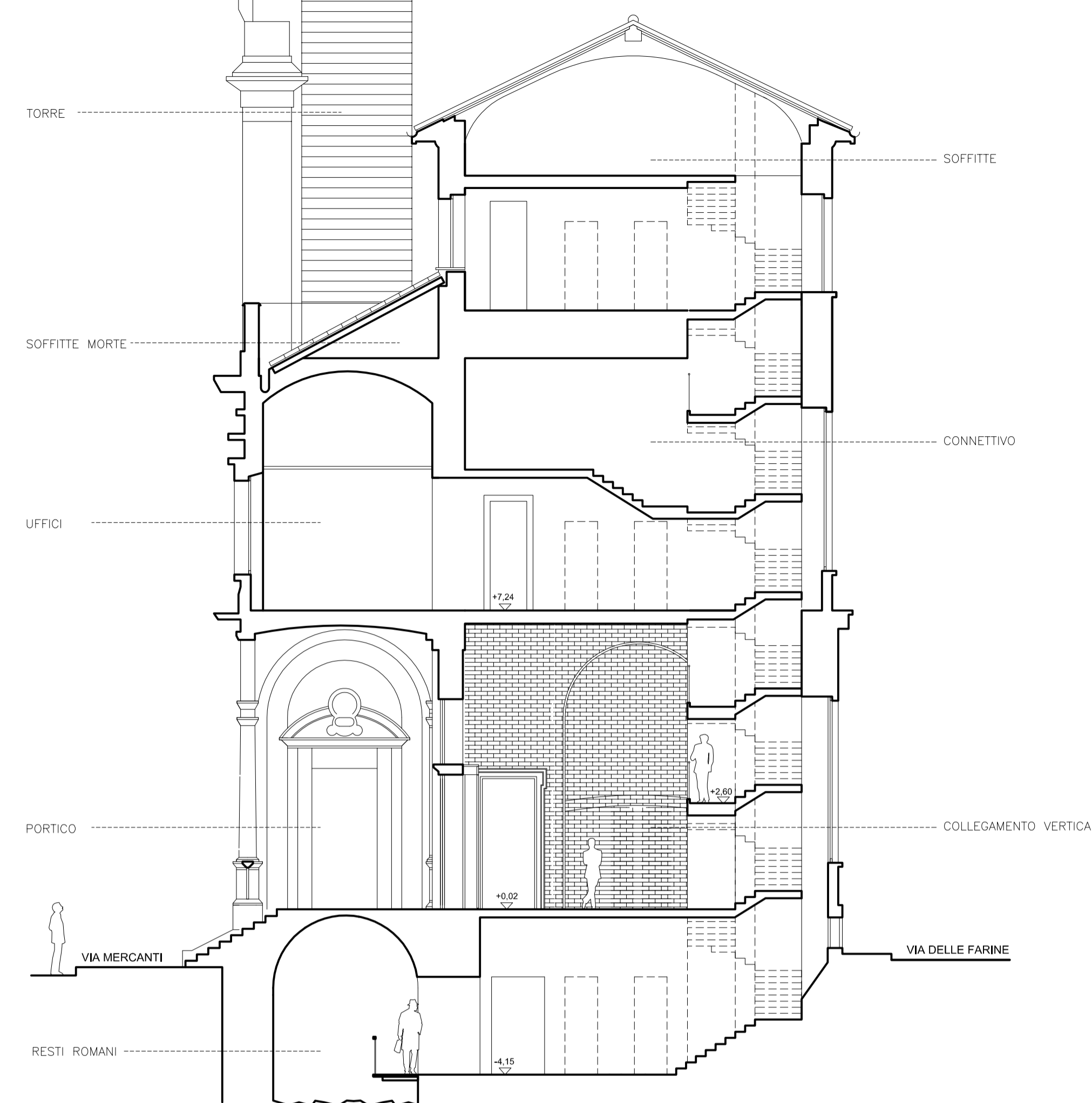
SEZIONE TRASVERSALE C-C
