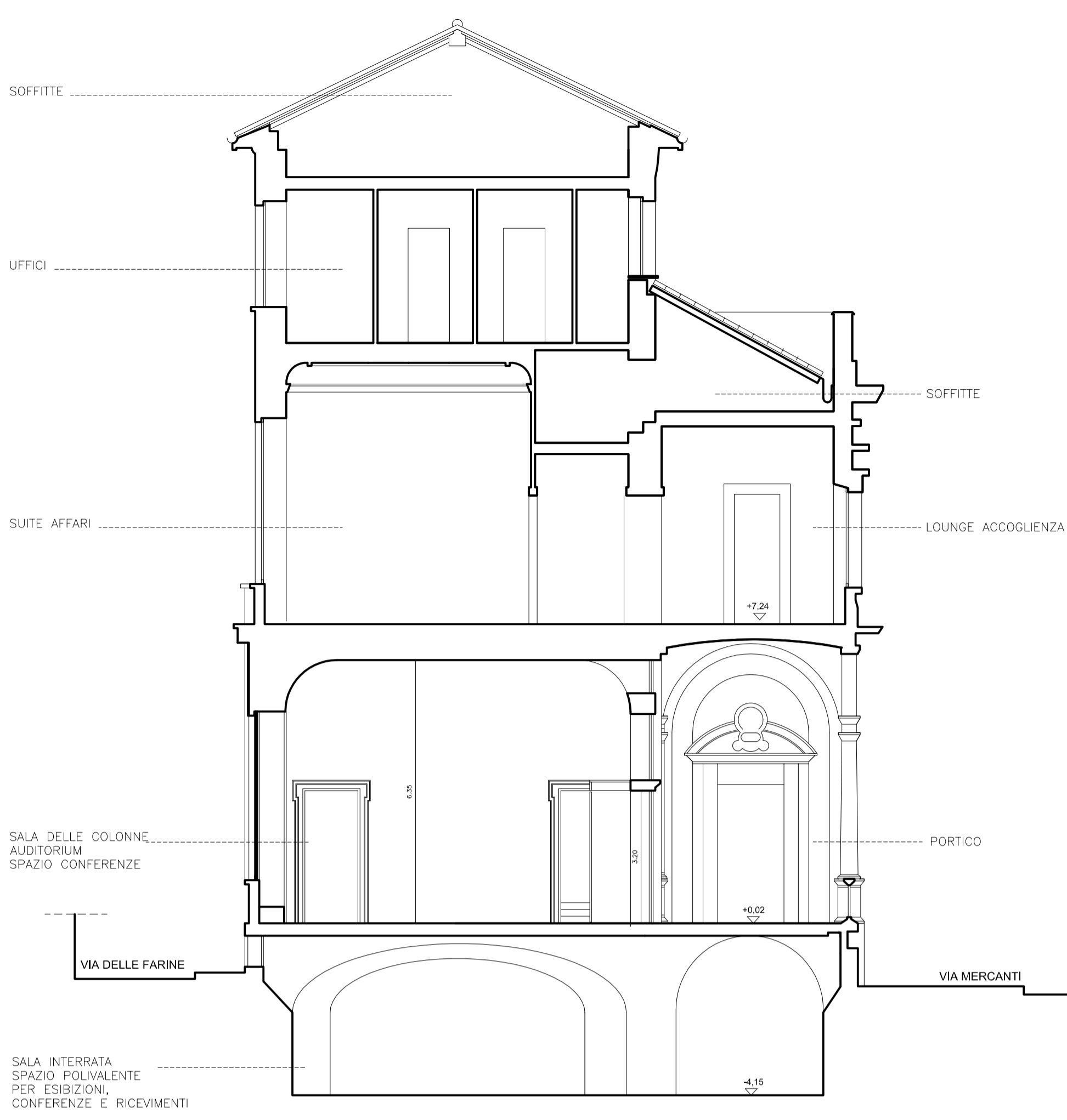
SEZIONE TRASVERSALE B-B
