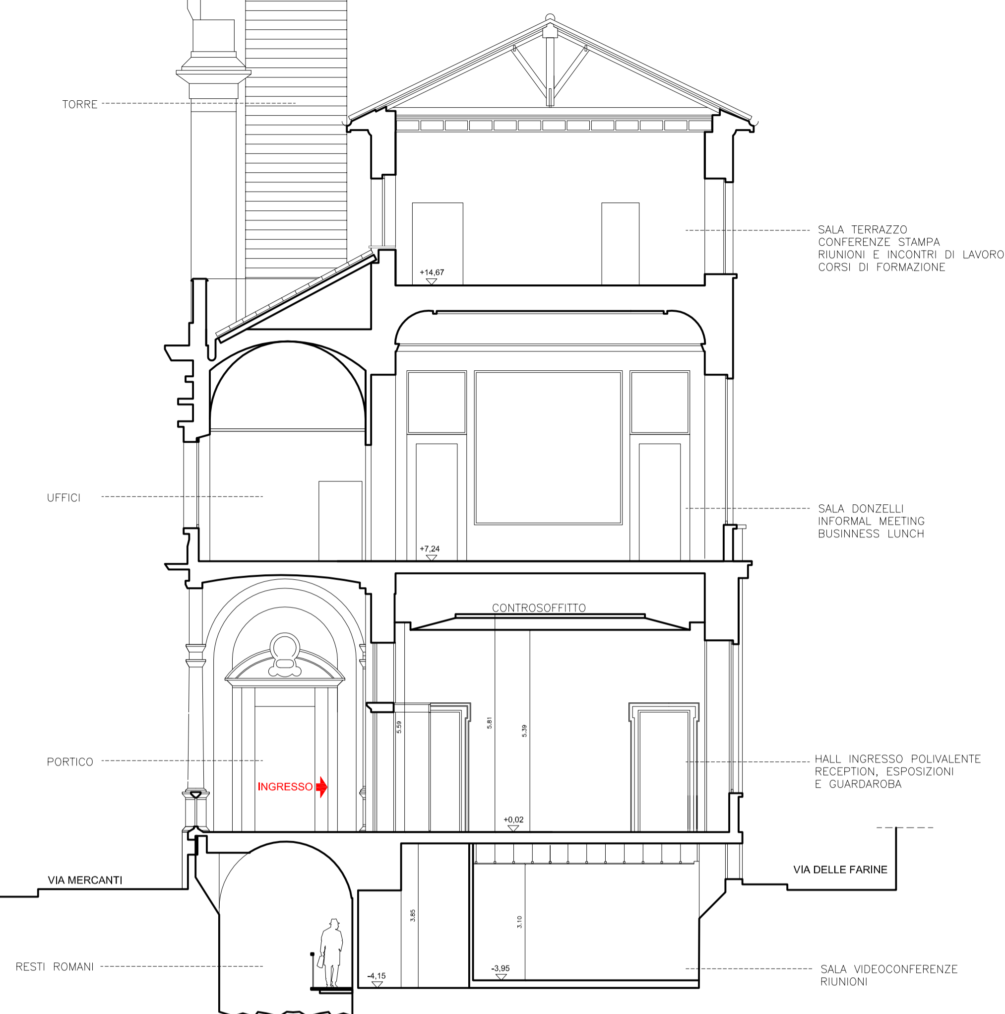
SEZIONE TRASVERSALE D-D
